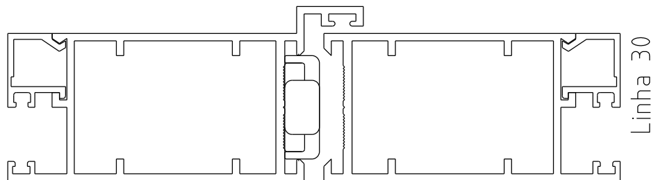
Instalação - escala 1:1
