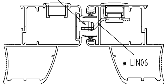
Instalação - escala 1:2
