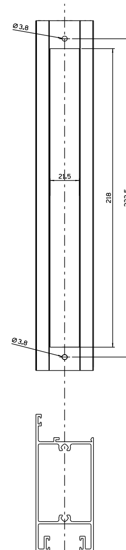
Usinagem - escala 1:2
