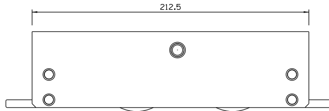
Vistas - escala 1:2
