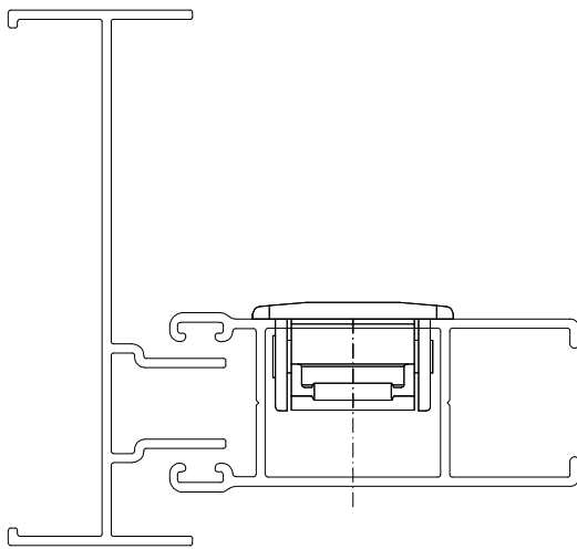
Instalação - escala 1:1
