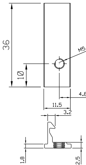
Vistas - escala 1:1
