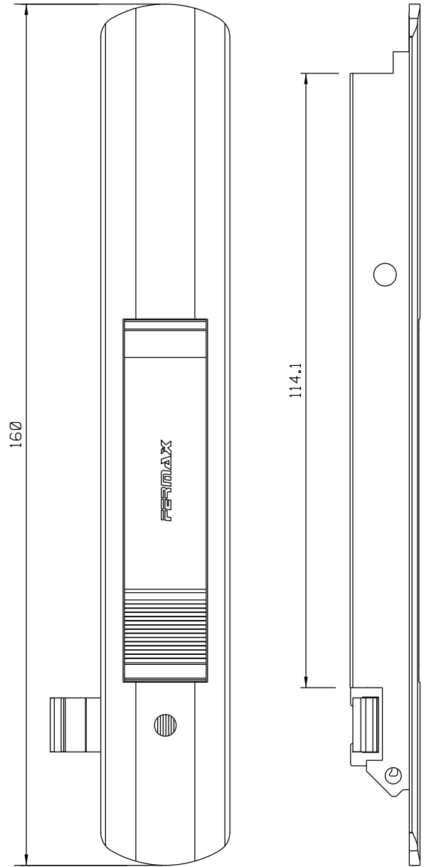
Vistas - escala 1:1
