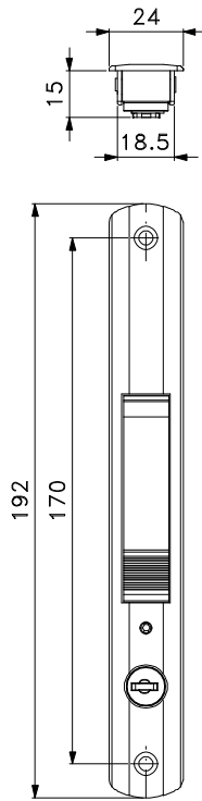
FEC 131 FEC 132
