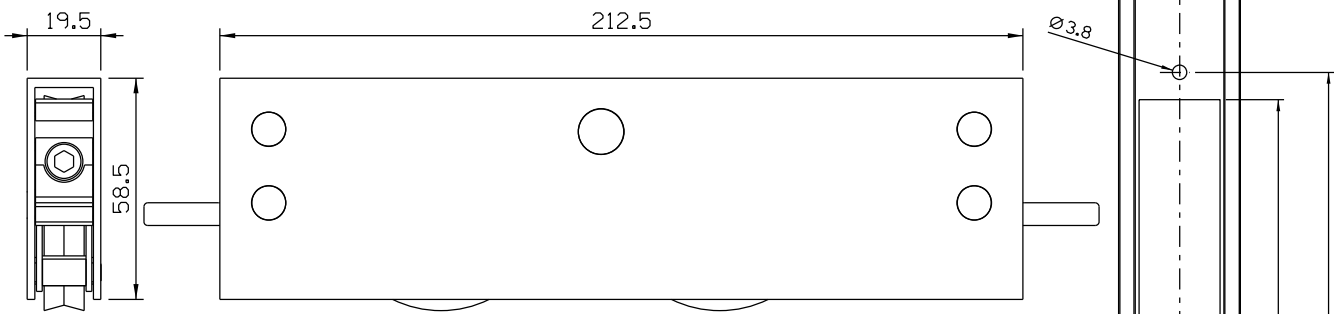
Vistas - escala 1:2
