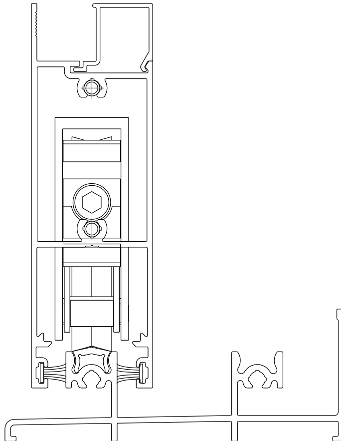
Vistas - escala 1:2
