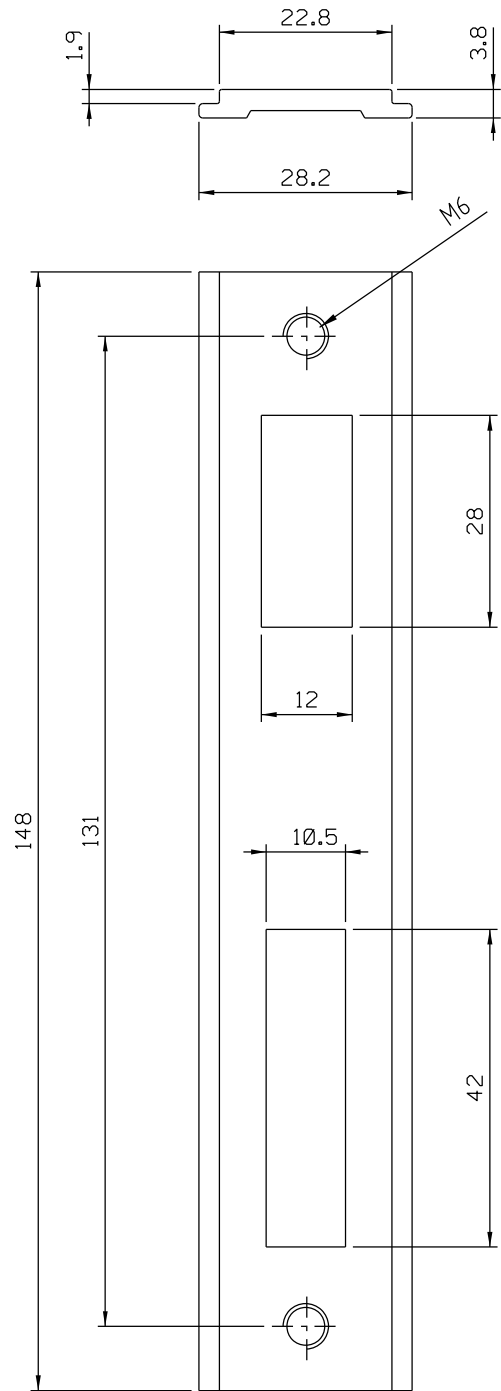
Vistas - escala 1:1
