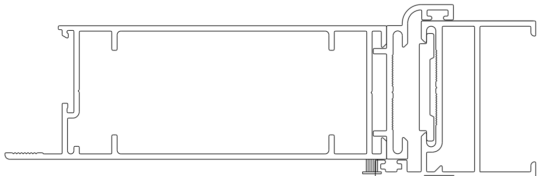
Vistas - escala 1:1
