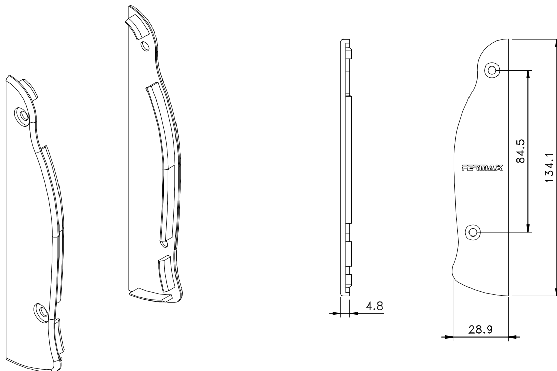
Vistas - escala 1:2
