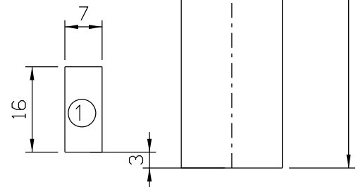
Usinagem - escala 1:1
