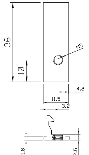
Vistas - escala 1:1
