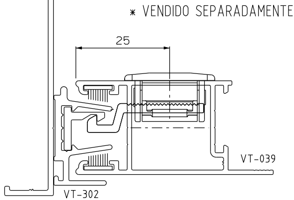
Instalação escala 1:1
