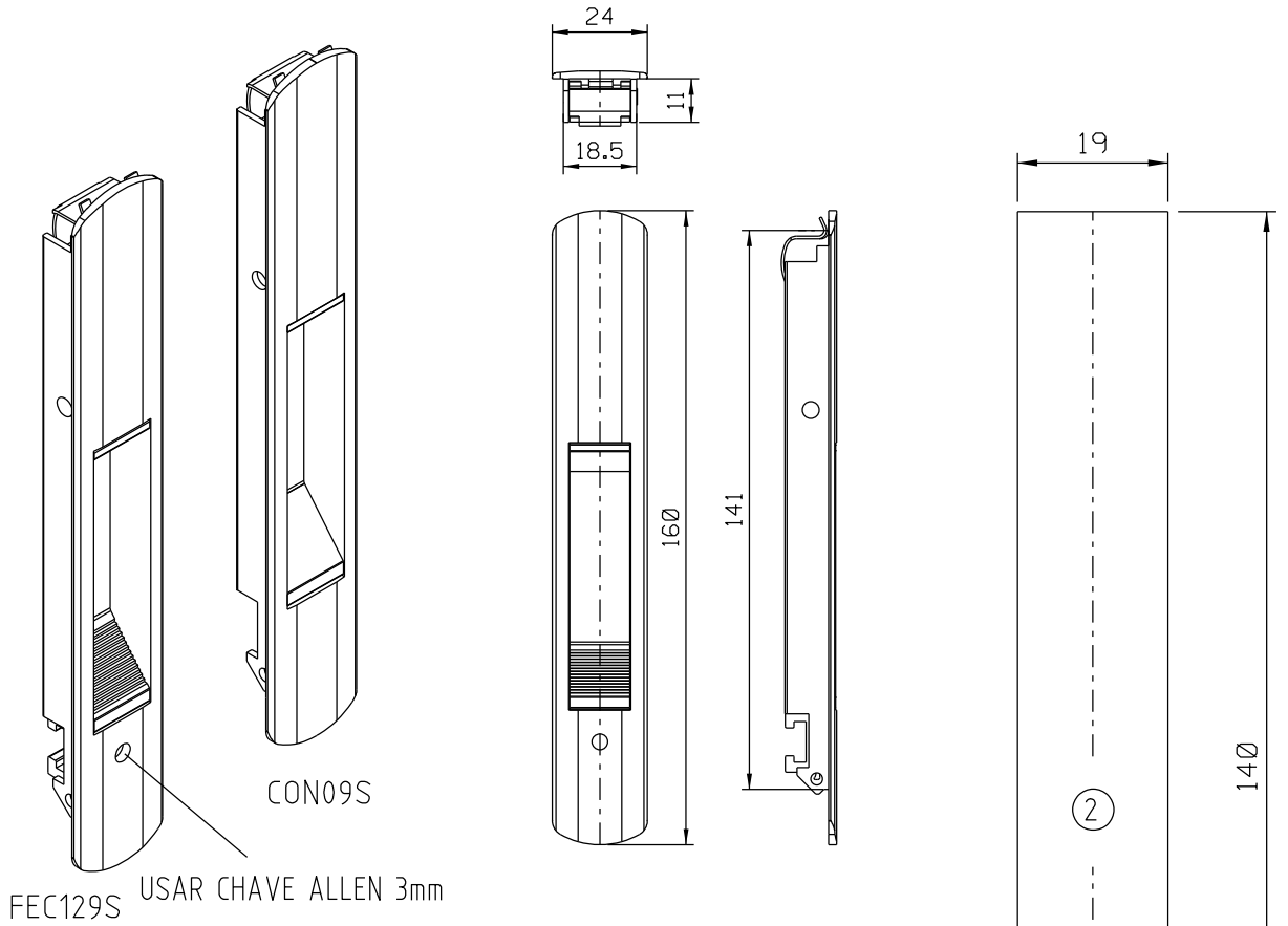
Vistas - escala 1:2
