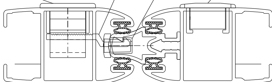
INSTALAÇÃO 1:1
