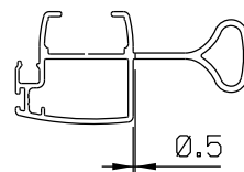
Vistas - escala 1:2
