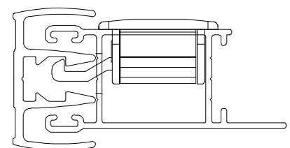
Vistas - escala 1:1
