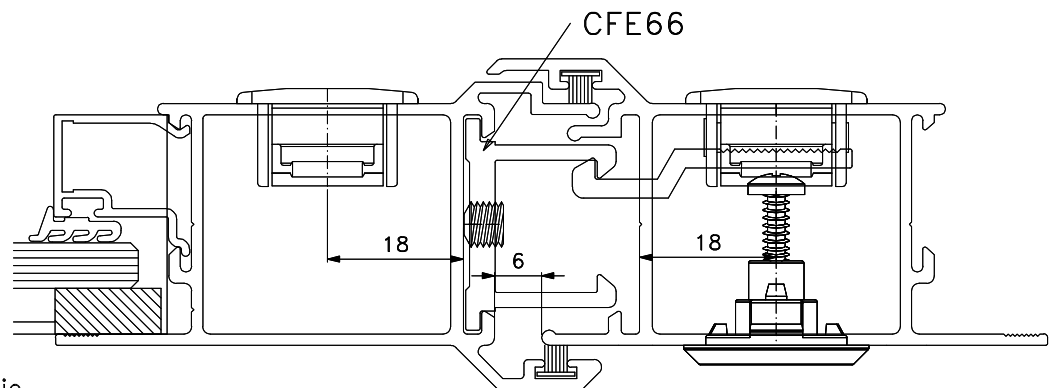
Instalação escala 1:1
