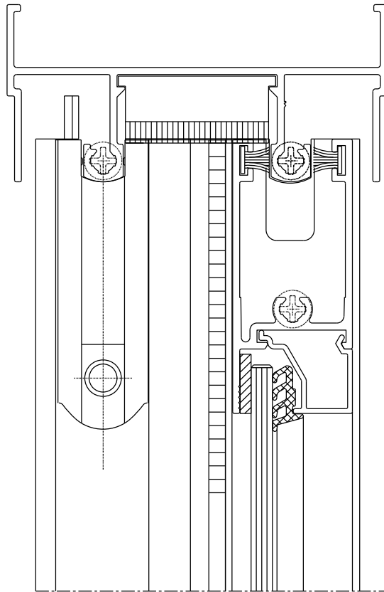
Instalação - escala 1:1
