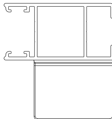
Instalação - escala 1:1
