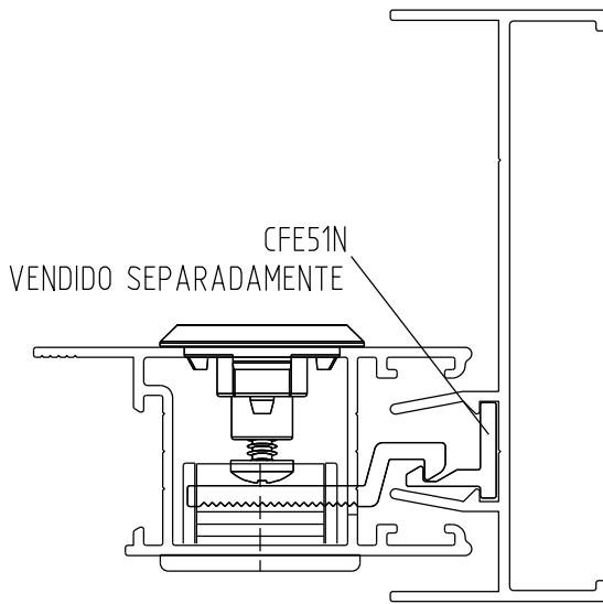
Instalação - escala 1:1
