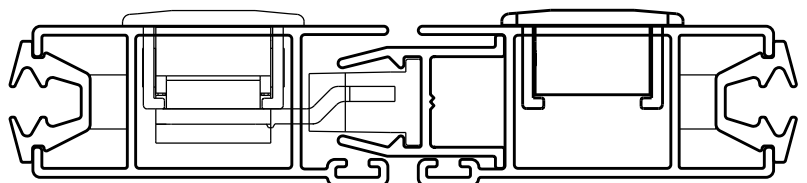
Instalação - escala 1:1
