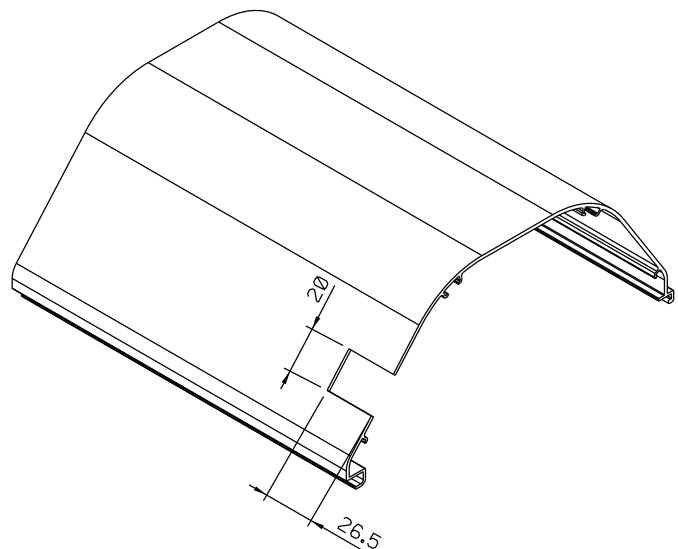
Vistas - escala 1:1
