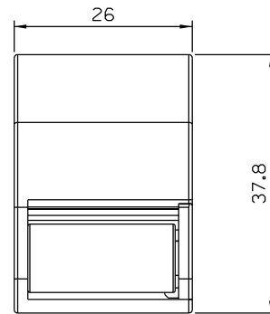
Vistas - escala 1:1
