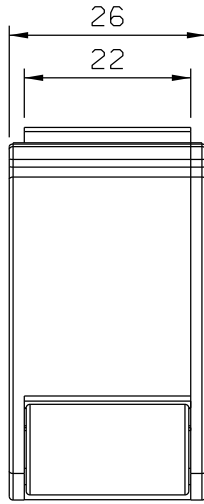
Vistas - escala 1:1
