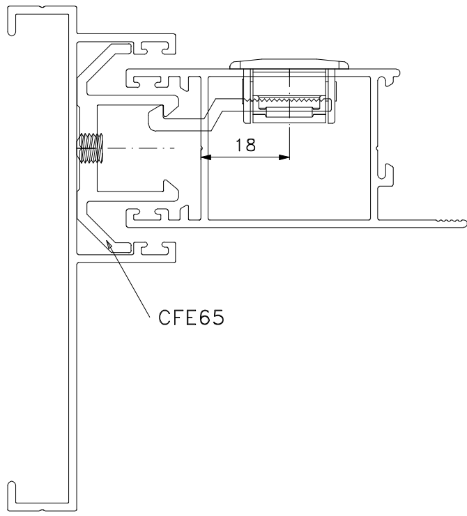
INSTALAÇÃO 1:1
