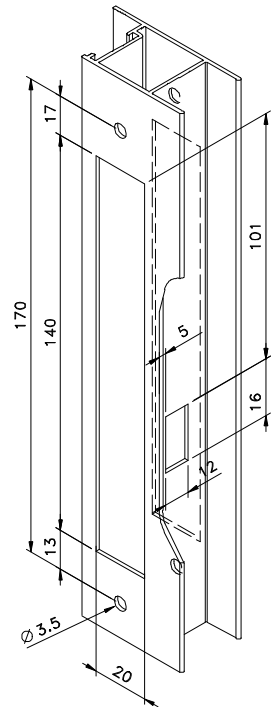
USINAGEM Sem escala
