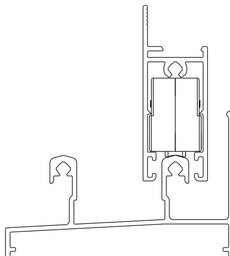
Instalação - escala 1:1
