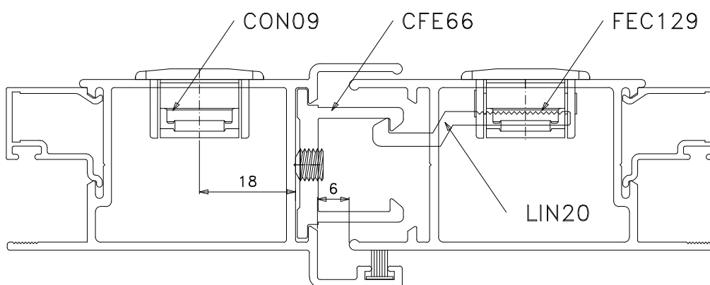
Instalação escala 1:1
