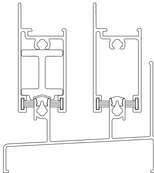
Instalação - escala 1:1
