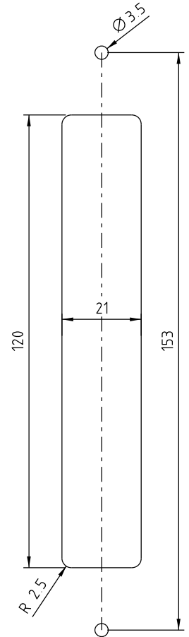
USINAGEM ESCALA 1:1
