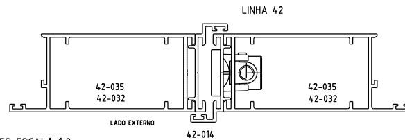
APLICAÇÕES ESCALA 1:2
