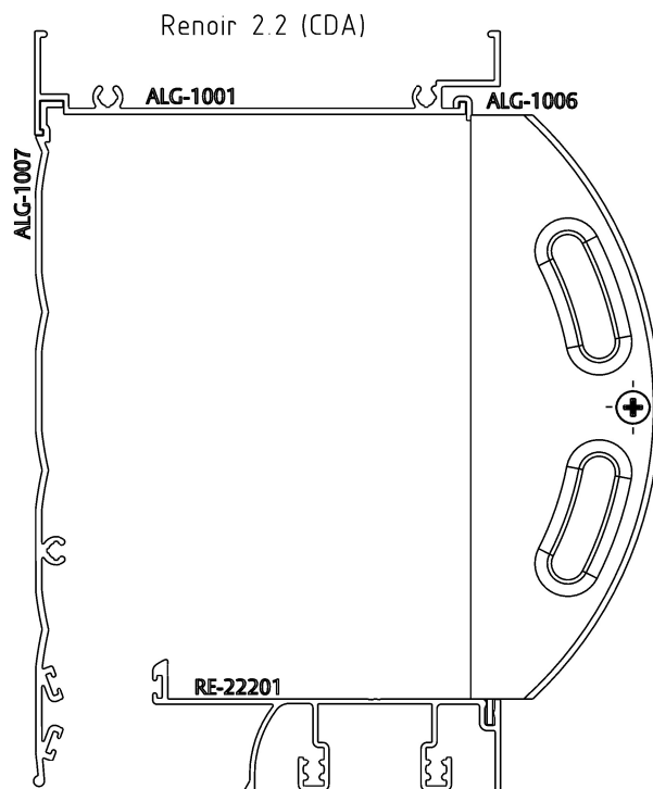
Instalação: escala 1:2
