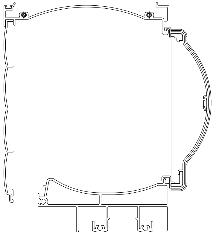
Instalação - escala 1:2
