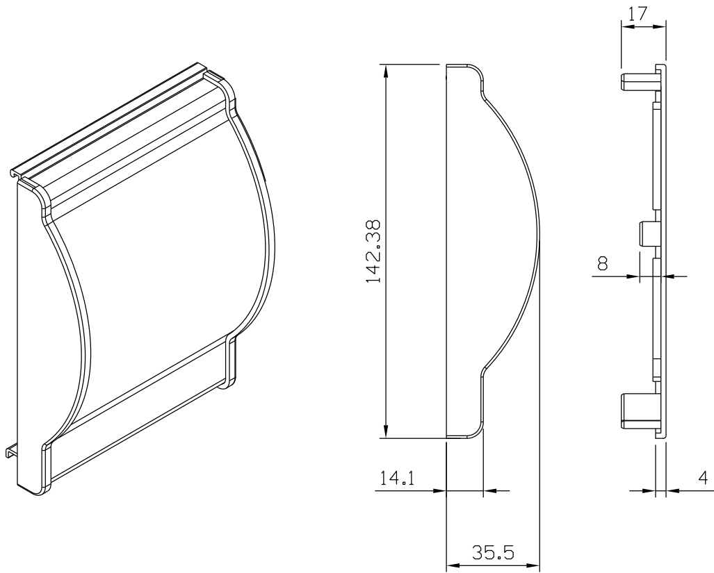
Vistas - escala 1:2
