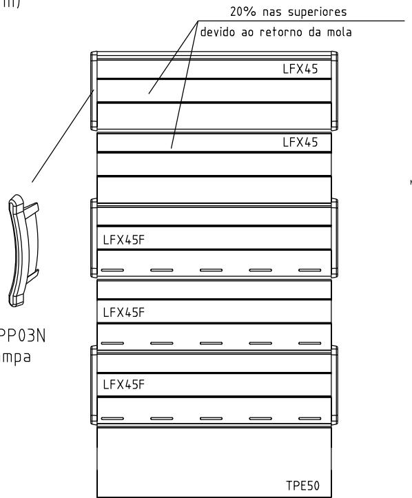
Orientação de montagem
