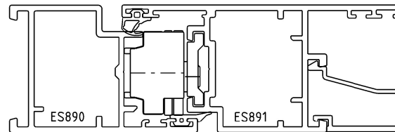
Instalação escala 1:1
