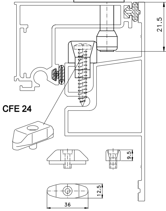
Contra-fecho - escala 1:2
