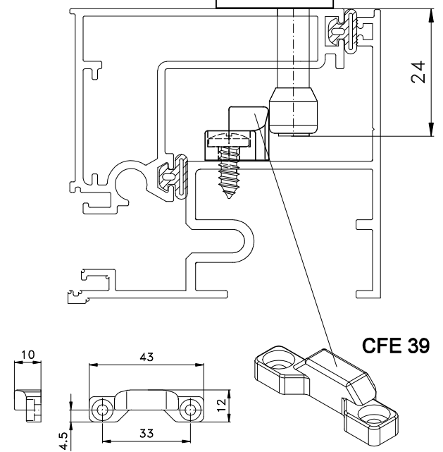
Contra-fecho - escala 1:2
