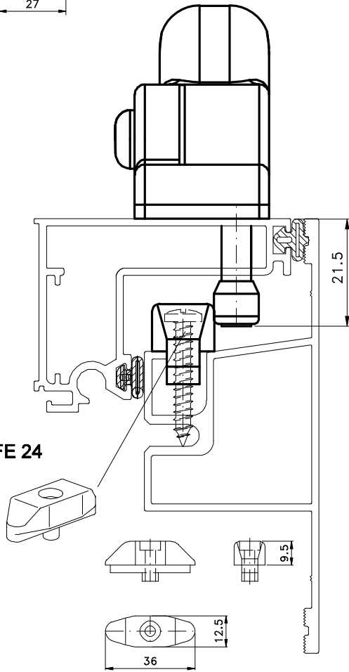
Contra-fecho - escala 1:2
