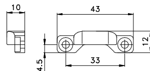
Contra-fecho - escala 1:2
