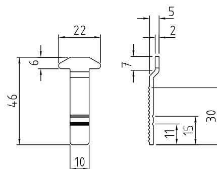
Vistas - escala 1:2
