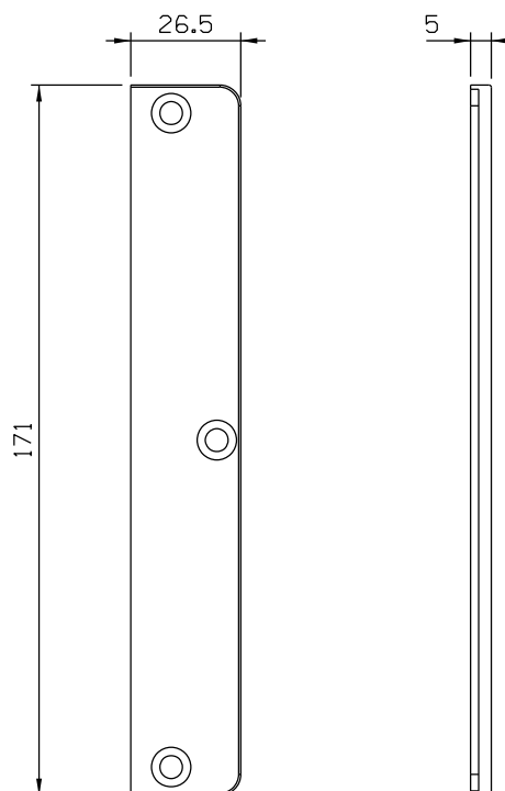
Vistas - escala 1:2
