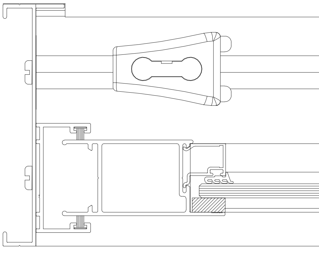
Vistas - escala 1:1
