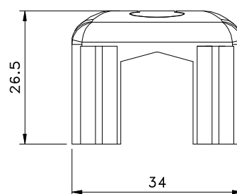
Vistas - escala 1:1
