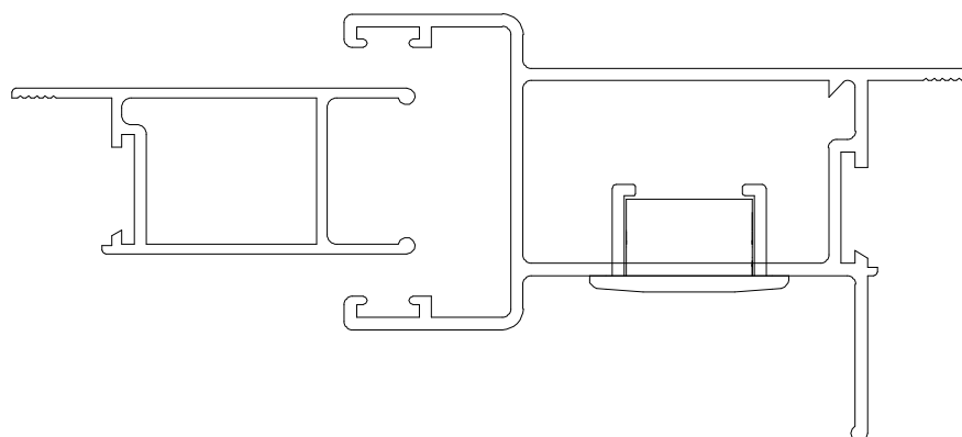
Instalação – escala 1:1
