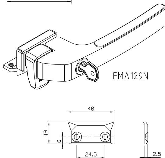
Contrafecho - Escala 1:2
