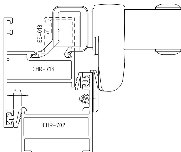
INSTALAÇÃO - ESCALA 1:1
