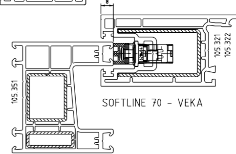
EKOLINE - VEKA
