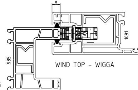
PREMILINE 58 - KOMMERLING
