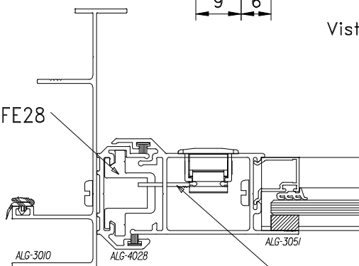
Instalação - escala 1:2
