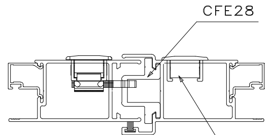
Usinagem para instalação Sem escala
