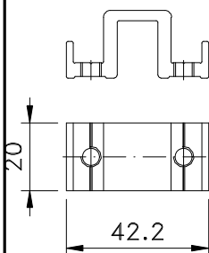
Vistas - sem escala
