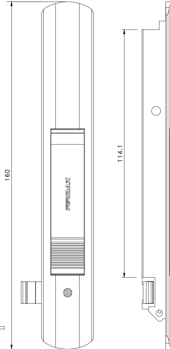
Vistas - escala 1:1
