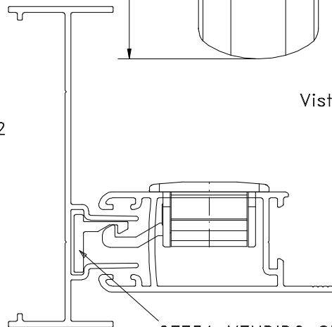
Instalação - escala 1:1
