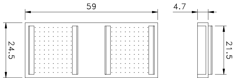
Vistas - escala 1:1
