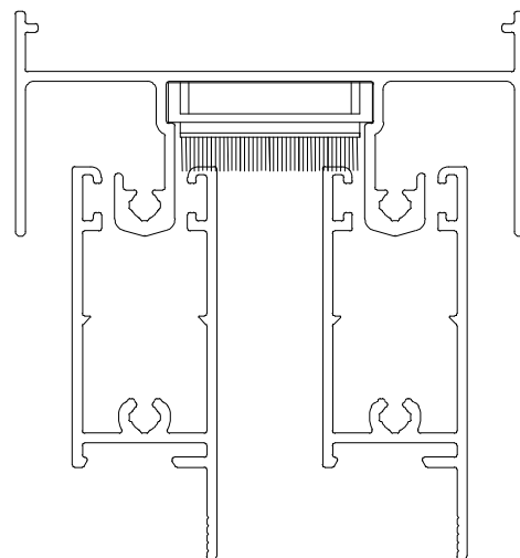
Instalação - escala 1:1
