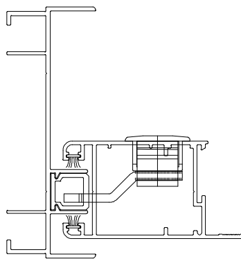
Vistas - escala 1:1
