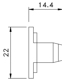
Vistas - escala 1:1
