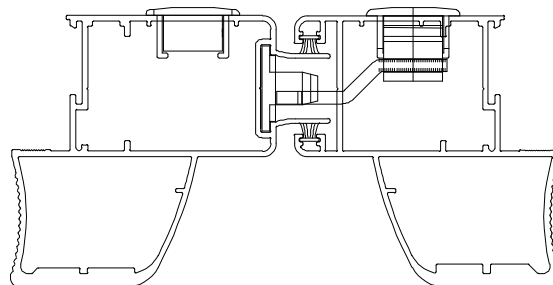
Instalação - escala 1:2
