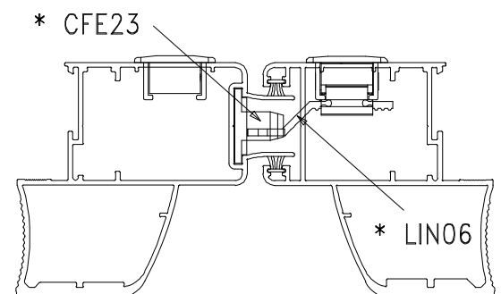
Instalação - escala 1:2
