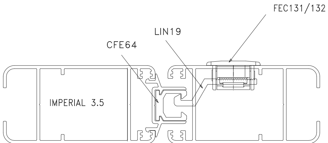
Instalação escala 1:1
