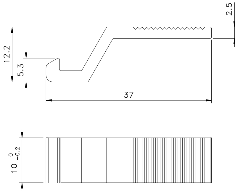
Vistas escala 2:1
