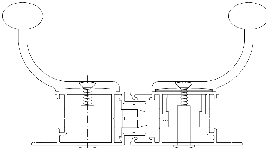
Instalação - escala 1:1
