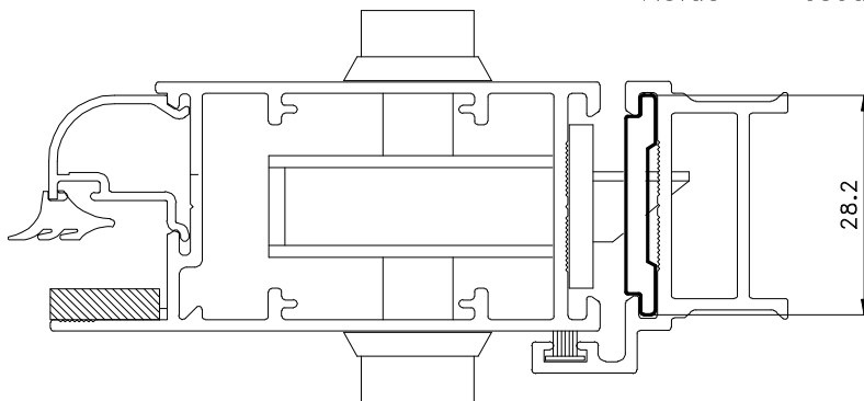
Vistas - escala 1:1
