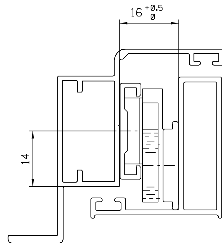
Instalação - escala 1:1
