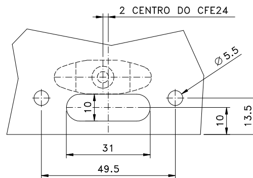
USINAGEM ESCALA 1:1
