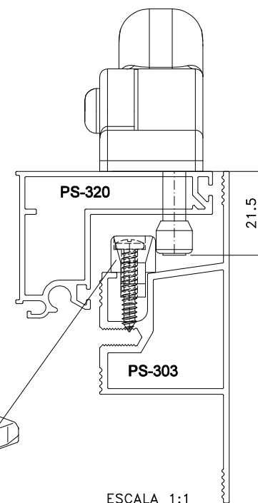
ESCALA 1:1
