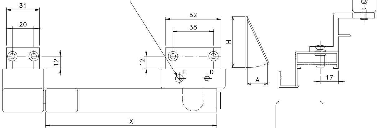
Vistas - escala 1:2
