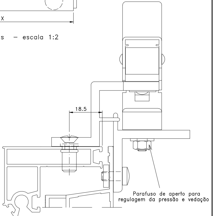
Instalação - escala 1:1
